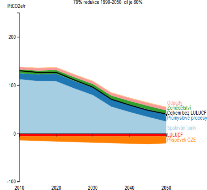
Emise skleníkových plynů 79% redukce 1990-2050; cíl je 80%
